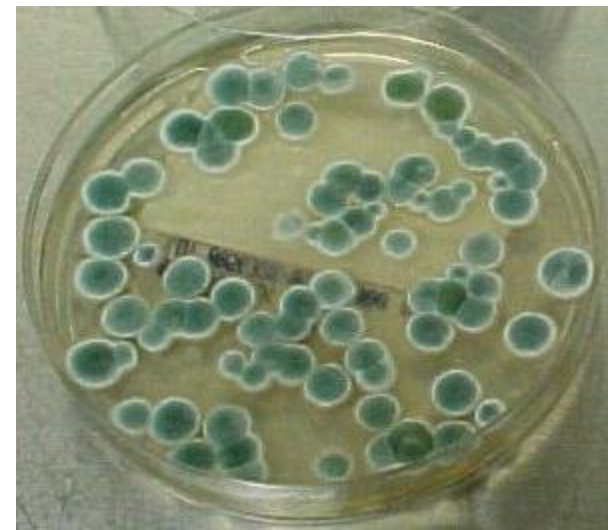
Cladosporium sp
