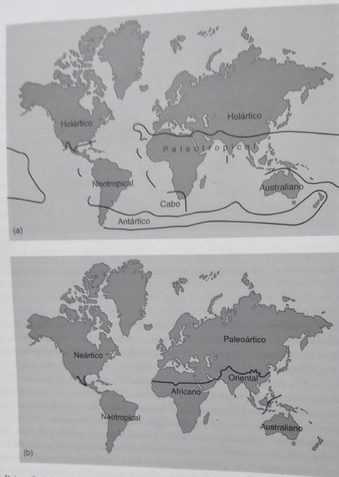
Fig. 2.2 (a) Reinos florísticos, segundo Good [11] e Takhtajan [12]. (b) Regiões zoogeográficas, segundo Selater [16] e Wallace [18]. Fonte: Cox [13].
